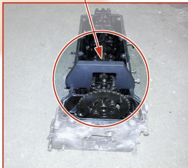
Nockenwellen-Einstellwerkzeug, BMW 11 3 190
