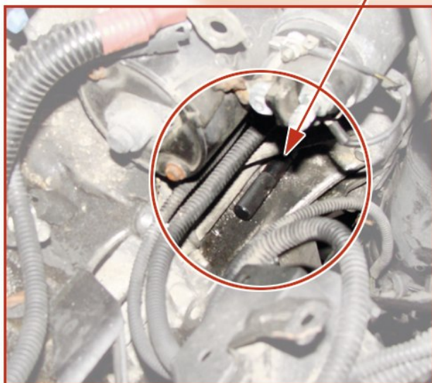
Schwungrad-Fixierdorn, BMW 11 2 300
