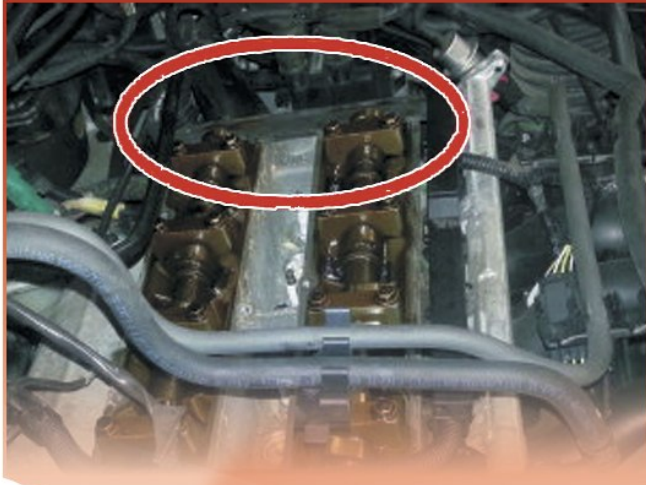
Kurbelwellenfixierdorn
